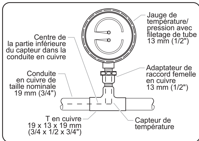
Installation alternative d'un indicateur de température/pression
