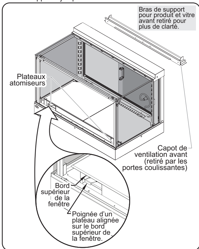
Vérification des plateaux atomiseurs (vue du IHDCH-45)
