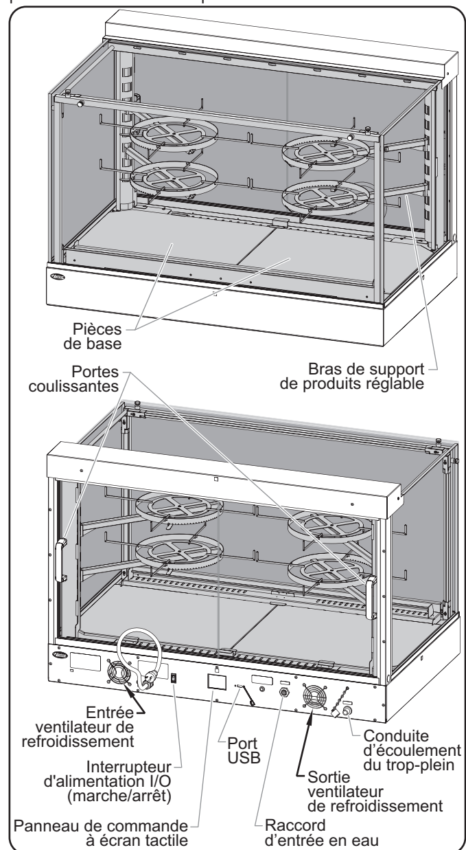
Vues avant et arrière du modèle IHDCH-45
