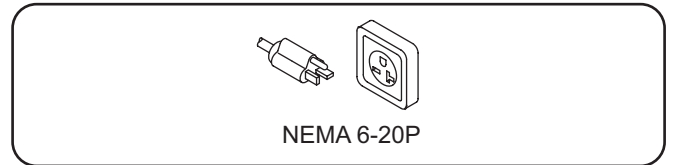
Configuration des fiches
