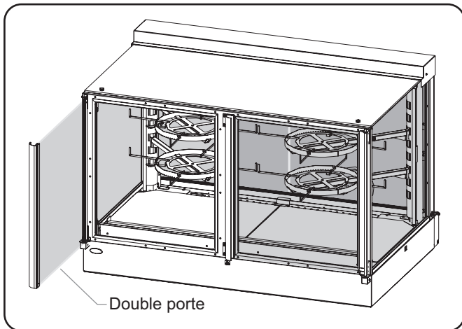
Double porte avant à fermeture automatique
