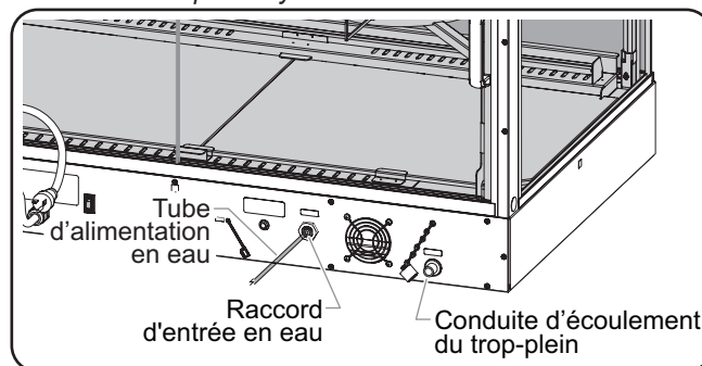
Raccordement de l'alimentation en eau (vue du IHDC-45)
